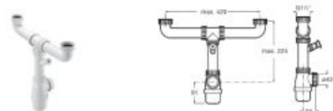
Sifón Blanco Para dos cubetas A506405507 € 16,50
