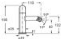
Grifería para bidé con cuerpo liso Con regulador de chorro a rótula y enlaces de alimentación flexibles. Maneta Dome
