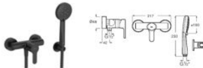
Grifería exterior para ducha Con ducha de mano Stella 100/3F, flexible 1,75m PVC satinado y soporte fijo Negro mate A5A2009NB4 € 183,00
