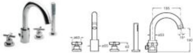
Grifería de repisa para baño- ducha Con caño central alto con inversor, ducha de mano y flexible de 1,75 m Cromado A5A0943C00 € 759,00
