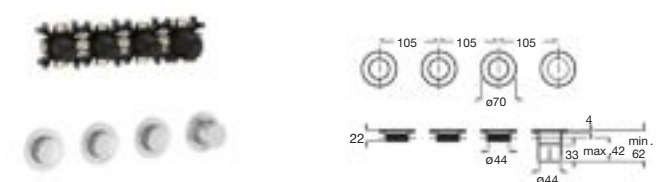
Grifería termostática empotrable 3 vías A completar con cuerpo empotrable
