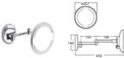
Espejo aumento pared x3 con luz LED, 2 brazos Cromado Ø210 A816380001 € 248,00
