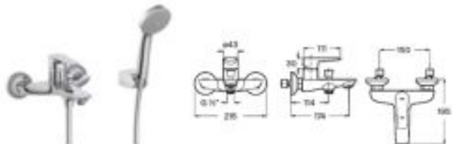
Grifería exterior para baño-ducha Con inversor automático con retención, ducha de mano Natura 80/1, flexible PVC de 1,7 m y soporte articulado
