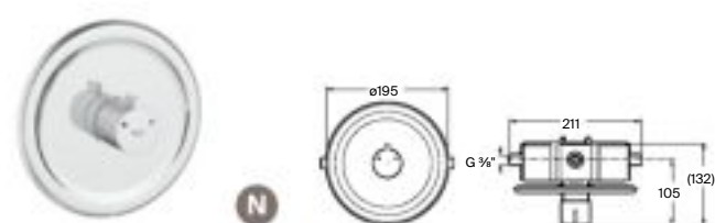
Grifería temporizada termostática empotrable para ducha Cromado Con rosetón Estándar A5A2579C00 € 451,00 Sist. Antilegionela A5A2G79C00 € 477,00
