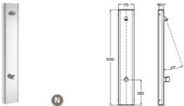
Panel de ducha temporizada en acero inoxidable con mezclador termostático Mezclador A5A2679C00 € 1.113,00
