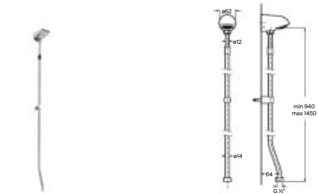
Conjunto de tubo, brida y rociador Cromado A5B9979C00 € 196,00
