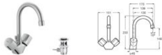
Grifería para lavabo Con aireador, caño giratorio, desagüe automático y enlaces de alimentación flexibles
