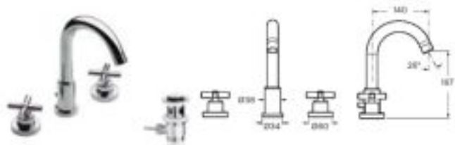
Grifería para lavabo Con caño central giratorio, aireador, desagüe automático y enlaces de alimentación flexibles Cromado A5A4443C00 € 523,00
