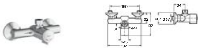
Grifería temporizada para ducha mural Cromado A completar con conjunto de tubo, brida y rociador A5B9979C00 A5A2D79C00 € 309,00
