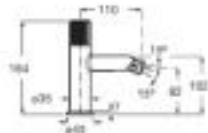
Grifería para bidé con cuerpo liso Con regulador de chorro a rótula y enlaces de alimentación flexibles. Maneta Stripes
