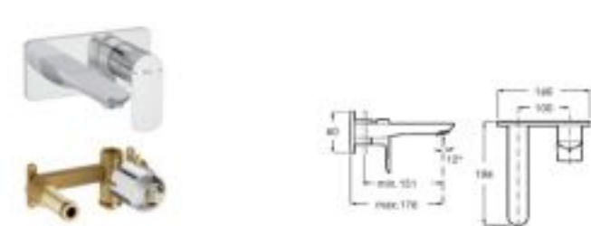
Grifería empotrable para lavabo A completar con cuerpo empotrable universal
