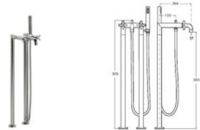
Grifería bimando de pie para baño- ducha Con inversor automático, ducha de mano, flexible de 1,75 m, soporte articulado y columnas verticales de alimentación Cromado A5A2743C00 € 1.459,00
