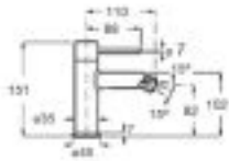
Grifería para bidé con cuerpo liso Con regulador de chorro a rótula y enlaces de alimentación flexibles. Maneta Pin
