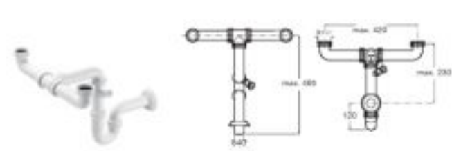
Sifón salvaespacio Blanco Para dos cubetas A506405707 € 18,50
