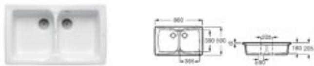
Beverly 85 Fregadero de dos cubetas, un orificio practicado y otro insinuado para la grifería y desagües de 3½" Blanco 860 x 500 x 205 A366057000 € 360,00
