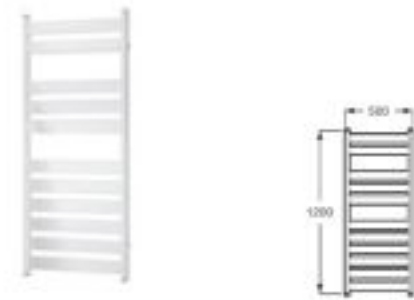
Toallero de agua Incluye kit de montaje, tapón y purgador 1200 Cromado A815509001 € 600,00 Blanco A815509000 € 445,00 Negro mate A815509NB0 € 488,00
