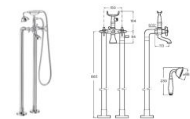
Grifería bimando de pie para baño-ducha Con inversor manual, ducha de mano, flexible de 1,50 m y columnas verticales de alimentación Cromado A5A274BC00 € 657,00
