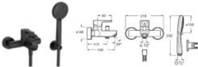
Grifería exterior para baño-ducha Con inversor automático con retención, ducha de mano Stella 100/3F, flexible 1,75m PVC satinado y soporte fijo Negro mate A5A0109NB4 € 209,00
