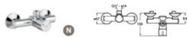
Grifería temporizada termostática para ducha mural Cromado A completar con conjunto de tubo, brida y rociador A5B9979C00. A5A2E79C00 € 351,00
