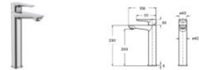
Grifería para lavabo de caño alto y cuerpo liso Con aireador y enlaces de alimentación flexibles
