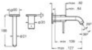
Grifería empotrable para lavabo Maneta Pin. A completar con cuerpo empotrable ref. A5E3502..0
