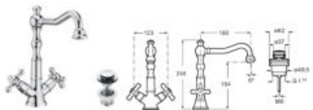
Grifería para lavabo con caño alto y cuerpo liso Con caño alto giratorio, aireador, desagüe click-clack y enlaces de alimentación flexibles Cromado A5A384BC00 € 231,00
