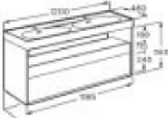
Mueble base para lavabo doble* Mueble base de dos cajones y estante abierto (lavabo no incluido)
